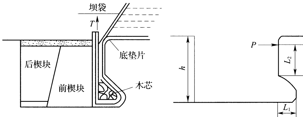
图 C. 2. 1 楔块锚固计算示意图
