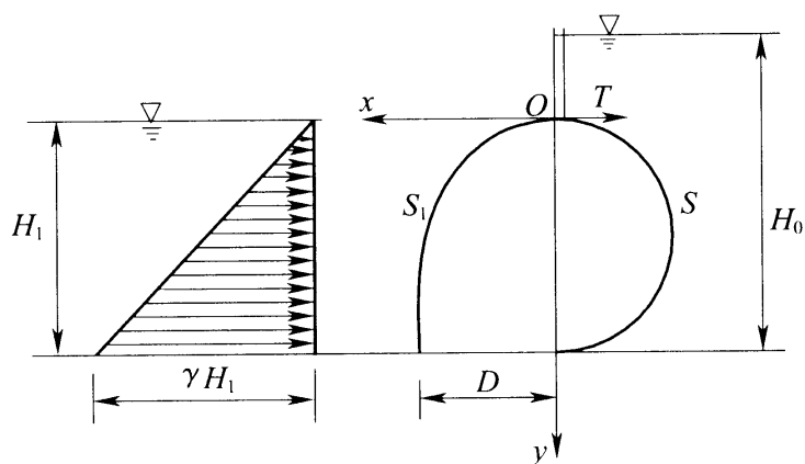
图 B. 3. 1 充气式橡胶坝示意图
