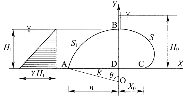
图 B.2.1 充水式橡胶坝示意图
