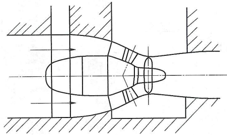
图 C.4 贯流式水轮机
