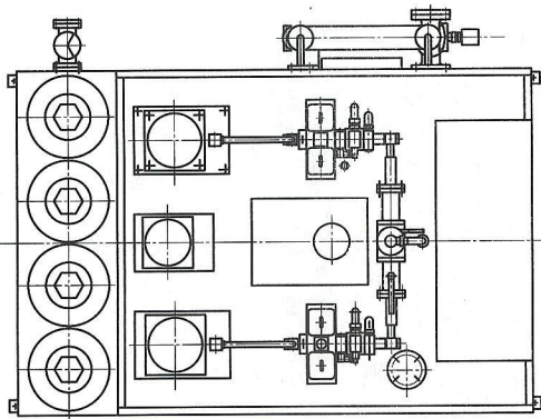
图 C.12 油压装置 (蓄能罐式)
