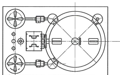
图 C.11 液压装置 (组合式)
