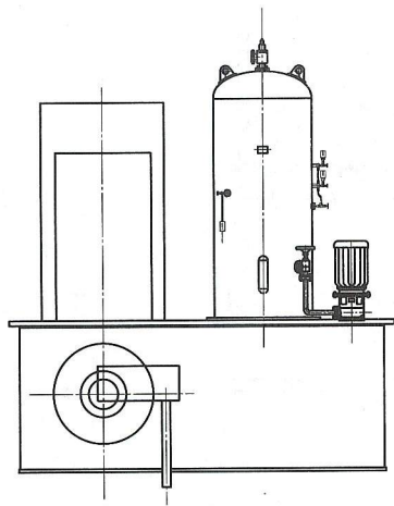
图 C.12 油压装置 (蓄能罐式)
