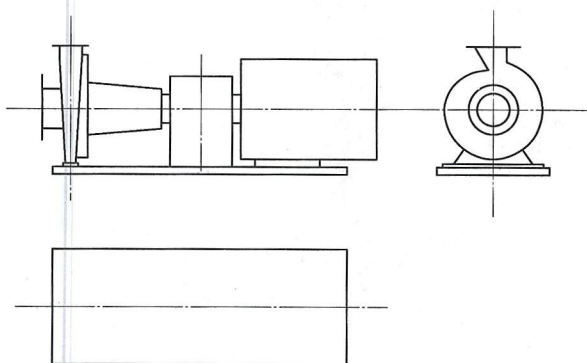
图 C.17 单吸离心泵
