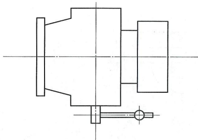
图 C.9 微阻缓闭止回阀
