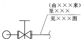
图 2.4.1 用文字表示的管路中断画法
