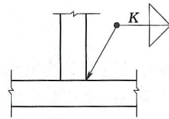
图 3.4.6 熔透角焊缝标注
