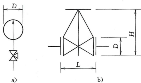
图 2.3.2-1 单线管路阀门、表的绘制
