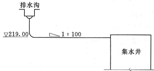
图 3.3.4-2 有坡度管路的标注
