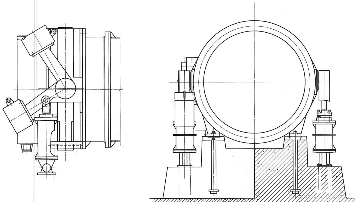
图 C.6 重锤式液压蝶阀
