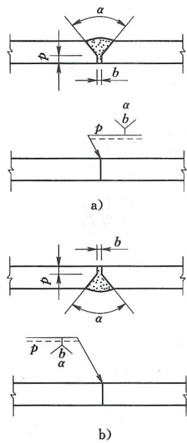
图 3.4.3 单面焊缝标注
