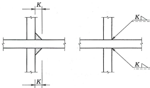
图 3.4.5-1 相互焊接焊缝标注
