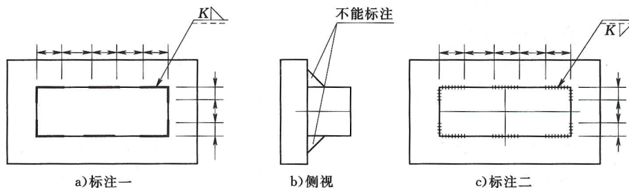
图 3.4.12 分布不规则的焊缝标注
