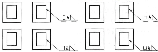
图 3.4.8 三面焊缝标注
