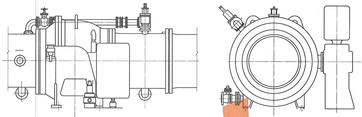
图 C.10 球阀
