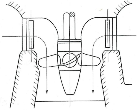
图 C.2 轴流式水轮机
