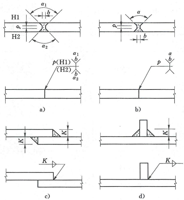
图 3.4.4 双面焊缝标注
