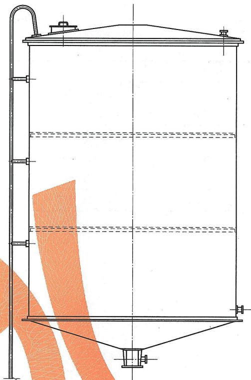
图 C. 26 油罐
