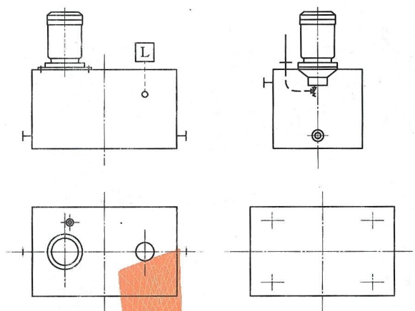
图 C. 21 漏油装置
