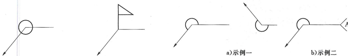
图 3.4.9 周围焊缝标注
