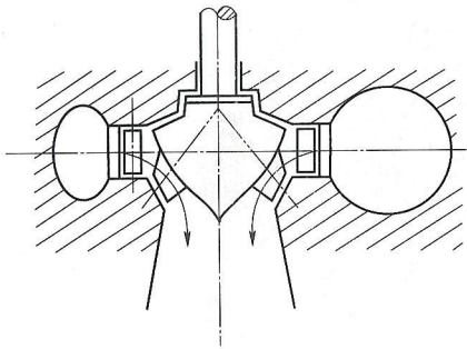
图 C.3 斜流式水轮机
