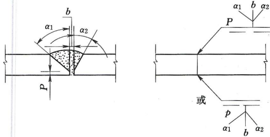
图 3.4.5-3 单面带双边不对称坡口焊缝标注
