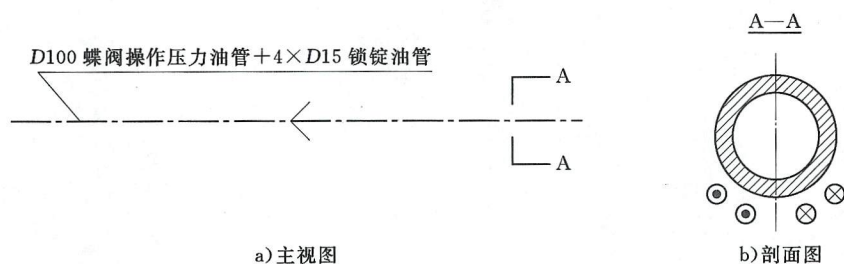
图 2.3.2-2 大直径管道上敷设小管的绘制
