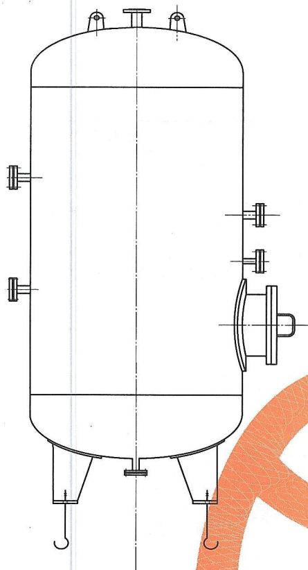
图 C. 25 气罐
