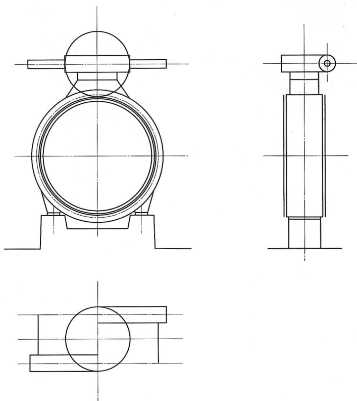
图 C.7 蝴蝶阀 (立轴式)
