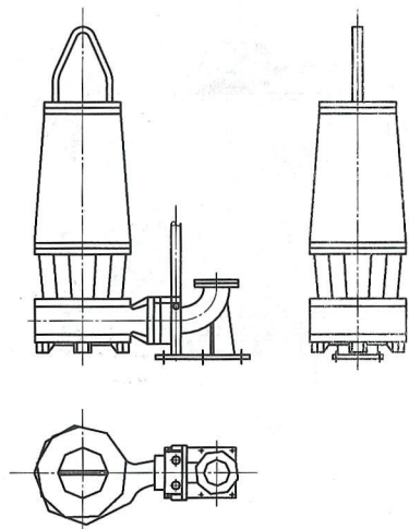
图 C. 20 潜水泵
