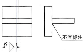
图 3.4.7 局部焊缝标注
