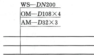
图 3.3.2 管路直径标注
