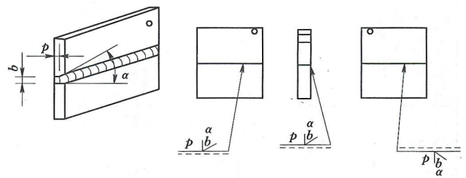
图 3.4.5-2 一个焊件带坡口时相互焊接焊缝标注
