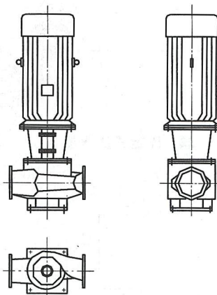
图 C.18 管道泵
