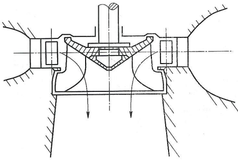
图 C.1 混流式水轮机
