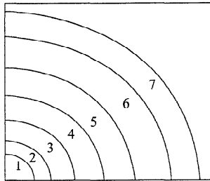
图 5.1.2-2 推移式连续浇筑施工
