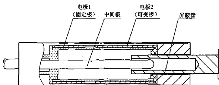
图 1 电容式位移计原理及结构示意图
