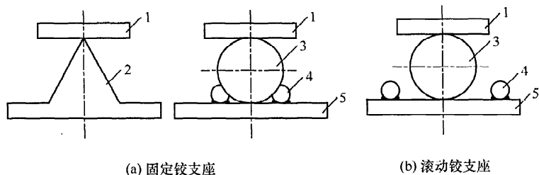
图 5.1.2-2 铰支座的形式
