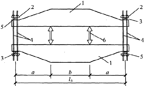
图 5.1.9 试件互为支座的对顶加载
