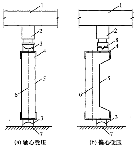
图 5.1.5-1 受压构件的支座布置
