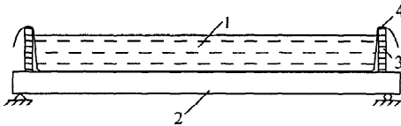
图 5.2.12 水压均布加载
