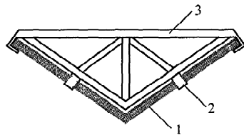
图 5.1.7 开口薄壁试件的定形架 1—薄壁构件；2—夹具；3—定形架
