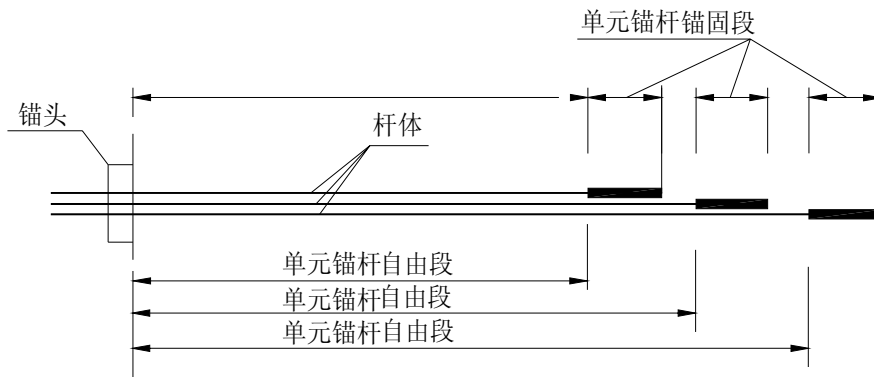
图 8 拉力分散型预应力锚杆结构示意图
