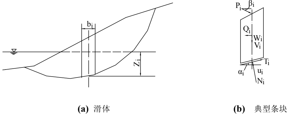
图 D.1.1 简化毕肖普法计算简图
