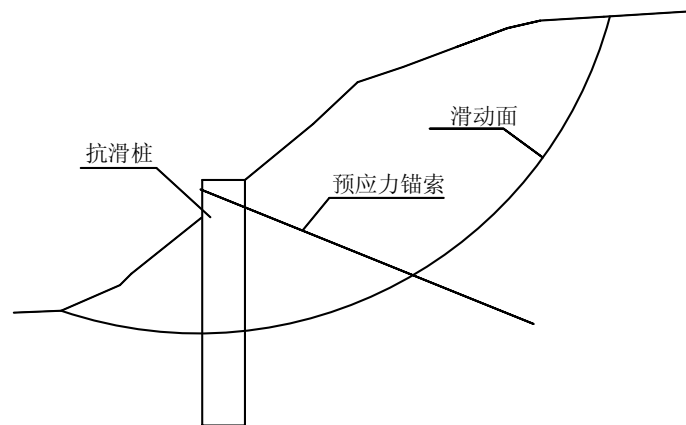
图 2 钢筋混凝土抗滑桩式锚杆挡墙
