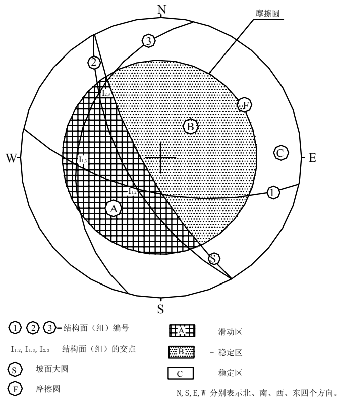
图 B.0.3 采用大圆分析法初步判别岩质边坡失稳可能性的极射赤平投影图
