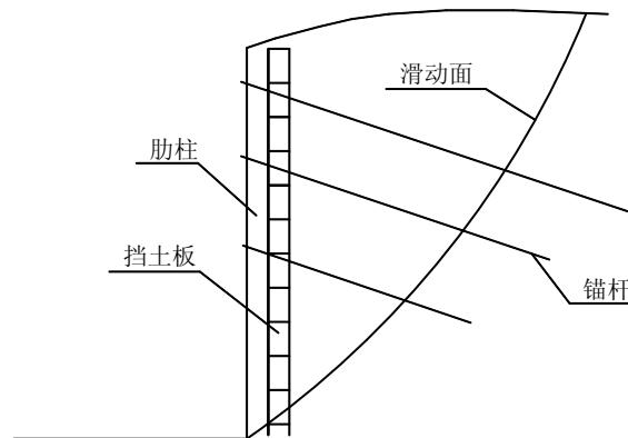
图4 钢筋混凝土板肋式锚杆挡墙
