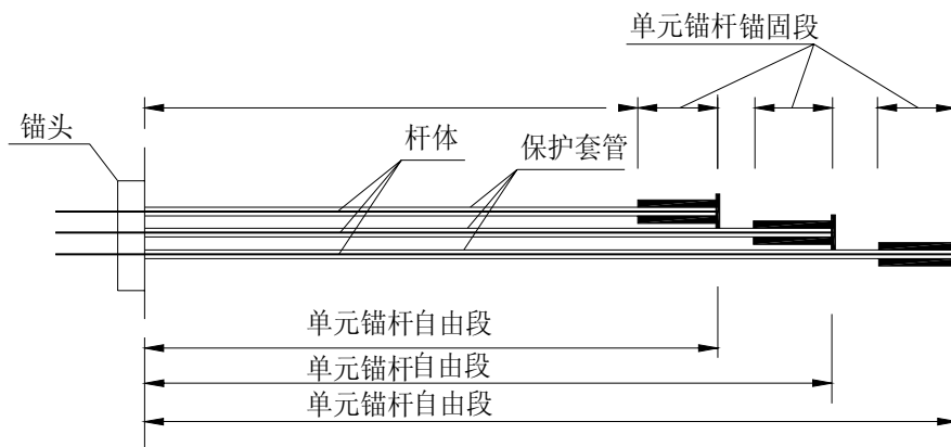
图 9 压力分散型预应力锚杆结构示意图
