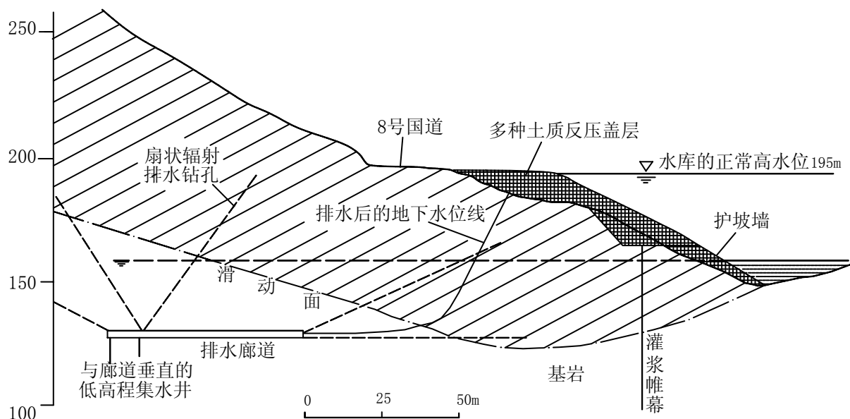
图 5 新西兰 Clyd 水电工程 Brewery Creek 滑坡加固工程
