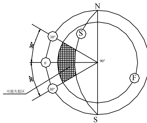
图 B.0.5 大圆分析法初步判别存在单组结构面的岩质边坡失稳可能性的极射赤平投影图
