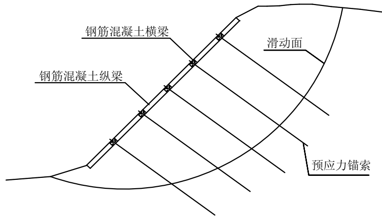
图3 钢筋混凝土格构式锚杆挡墙
