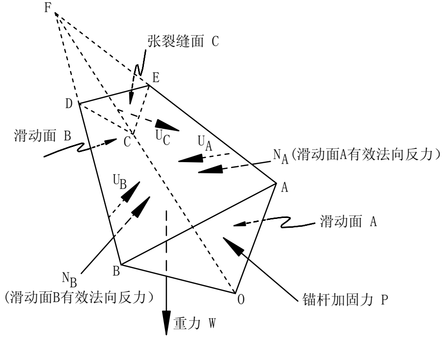
图 D.1.5 楔形体法计算简图
