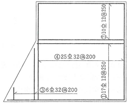
图 4.3.12 钢筋长度为等差时的简化标注
