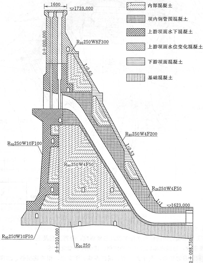
图 4.2.9-1 混凝土强度等级分区图
