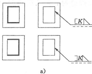
图 5.4.7 三面焊缝标注
