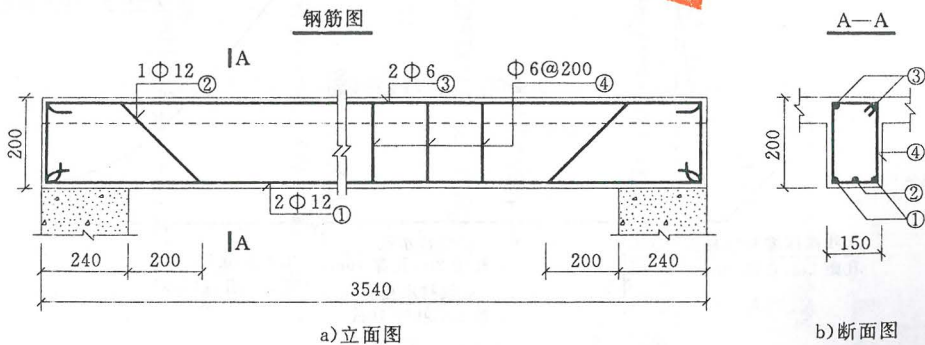
图 4.3.1 钢筋图
