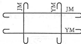
图 4.3.5-2 立面图中双层钢筋
