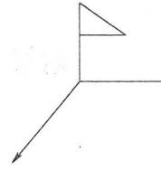
图 5.4.9 现场焊缝标注
