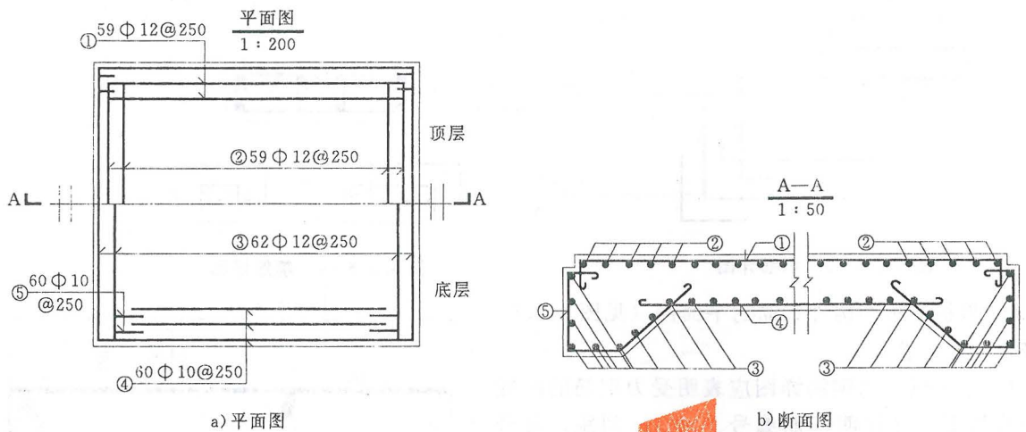
图 4.3.8 板类构件的面层和底层钢筋图
