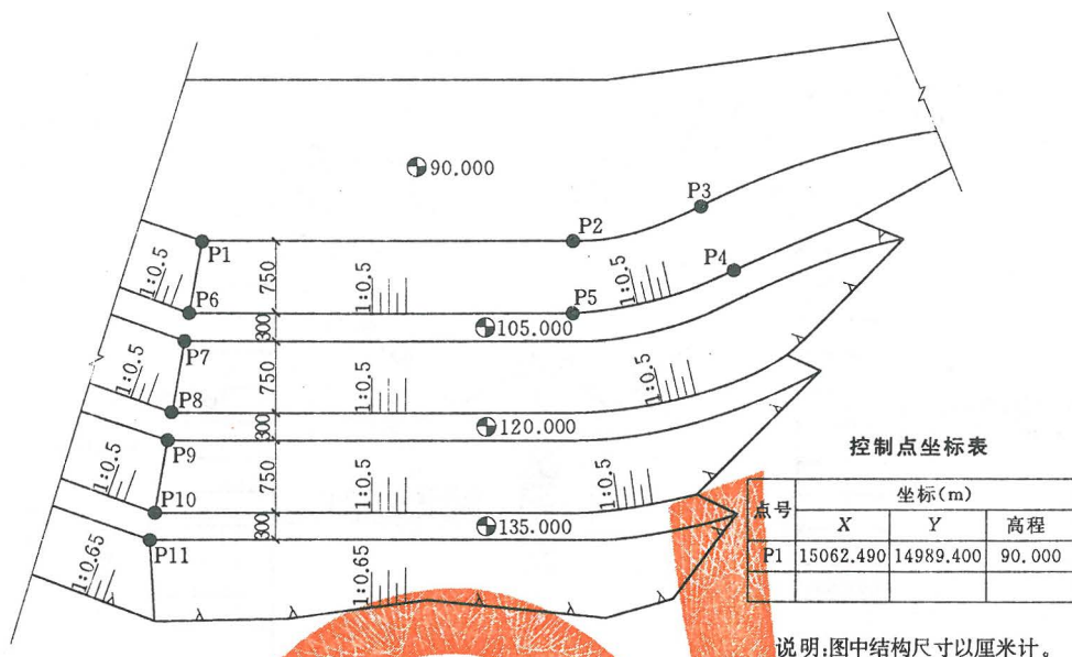
图 4.2.10-1 开挖平面图
