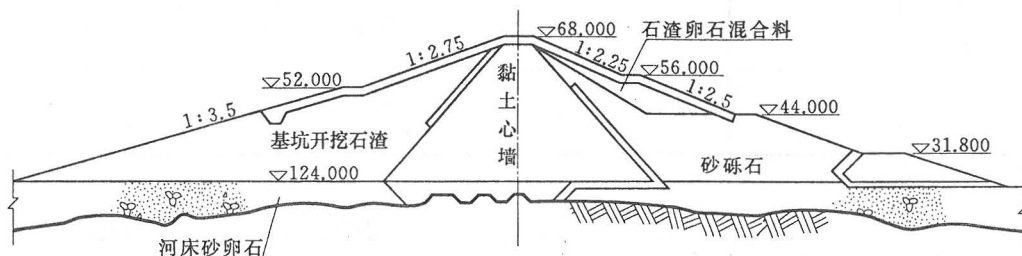
图 4.2.9-2 土石坝横断面图
