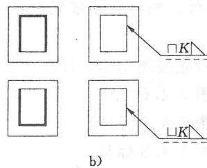
图 5.4.7 三面焊缝标注
