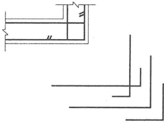
图 4.3.5-3 钢筋详图
