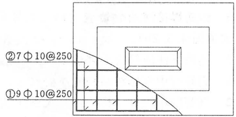
图 4.3.4-2 局部剖
