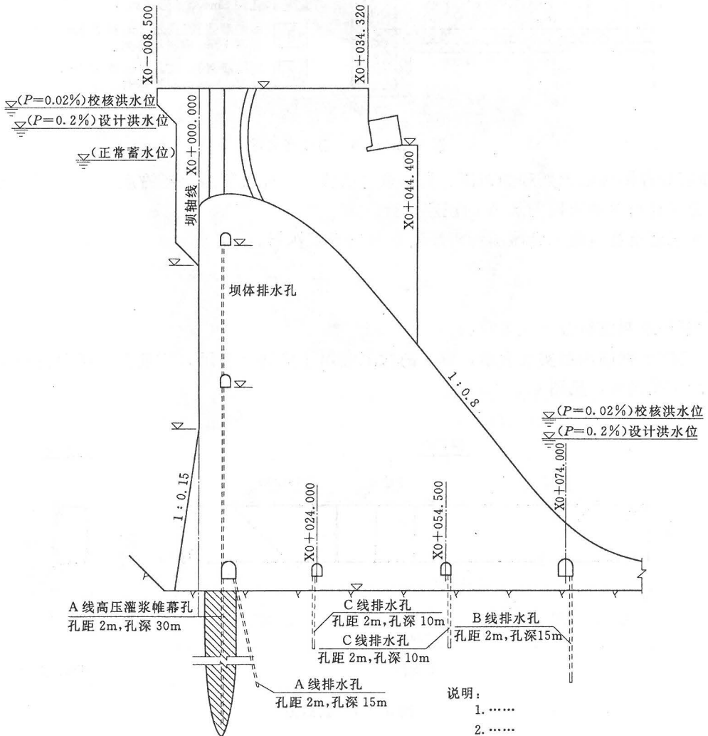
图 4.2.11-2 帷幕灌浆图
