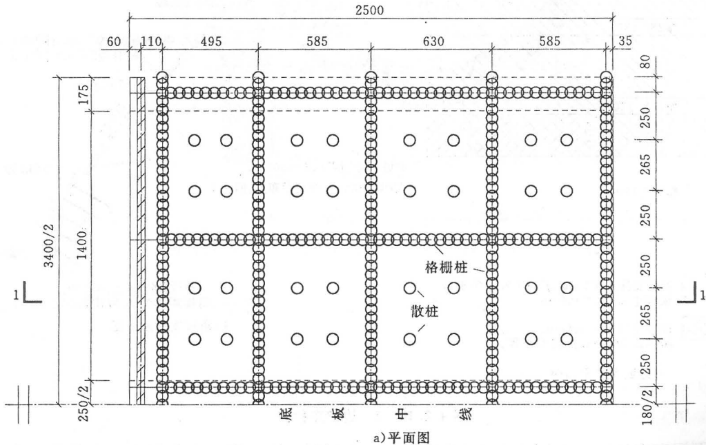
图 4.2.11-1 (一) 泄水闸软基处理图
