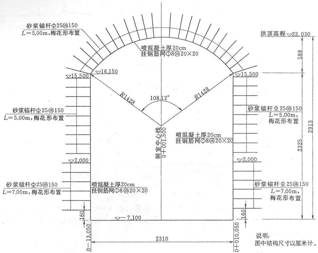
图 4.2.10-3 地下洞室支护图
