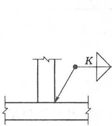
图 5.4.5 熔透角焊缝的标注
