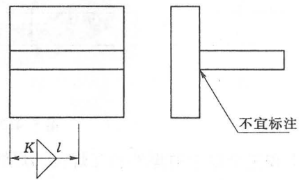
图 5.4.6 局部焊缝标注
