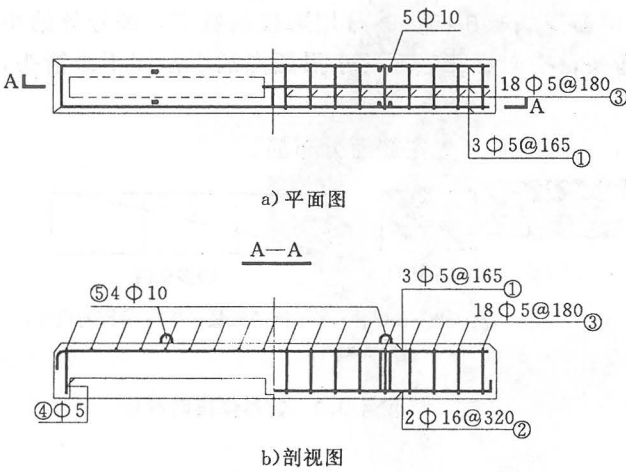
图 4.3.4-1 半剖及阶梯剖
