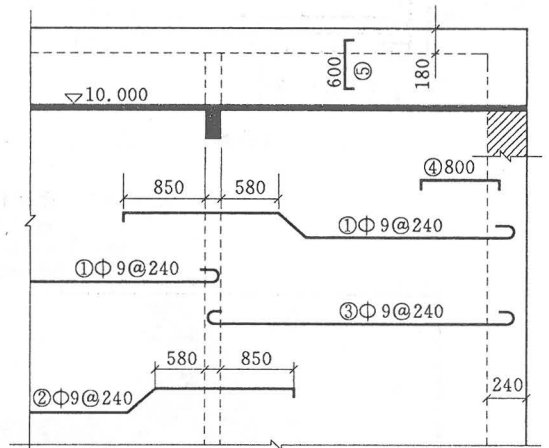
图 4.3.6 板类构件平面图中的钢筋表示法
