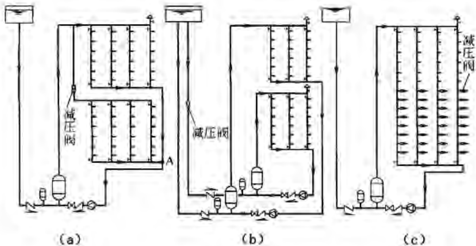
图3 减压阀设置
