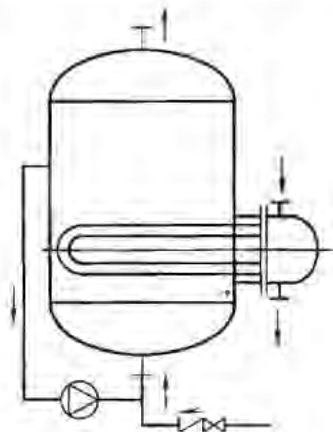
图 7 带外循环的容积式水加热器
