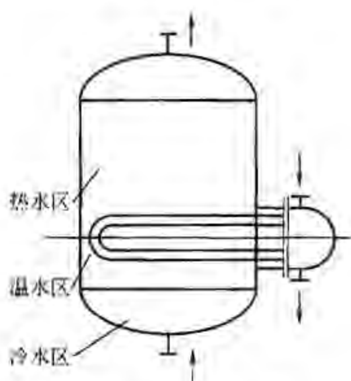
图5 容积式水加热器
