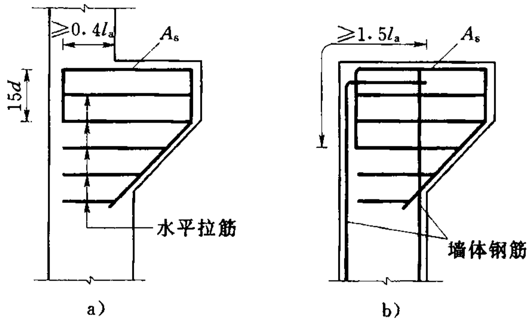
图 10.9.3 连续牛腿的配筋构造
