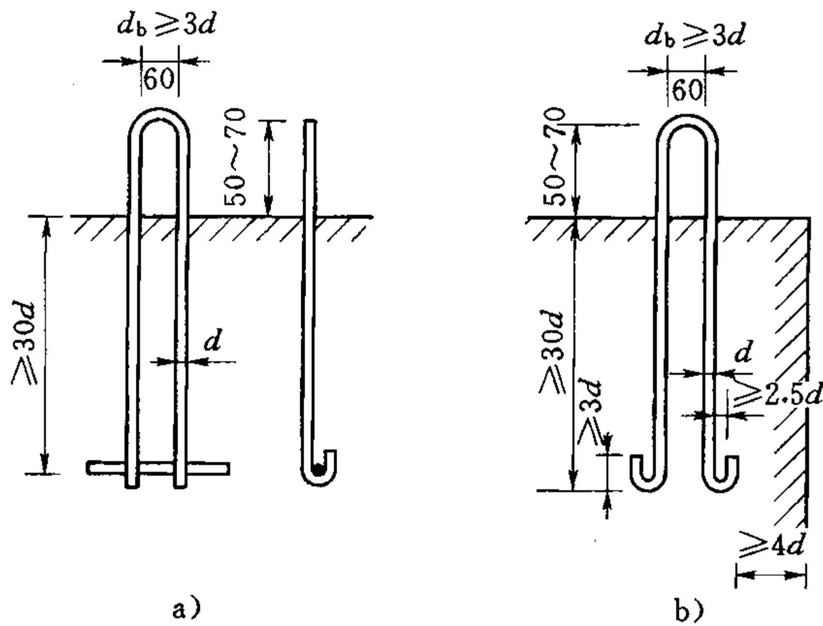
图 9.6.6 预制构件的吊环埋设 (单位: mm)
