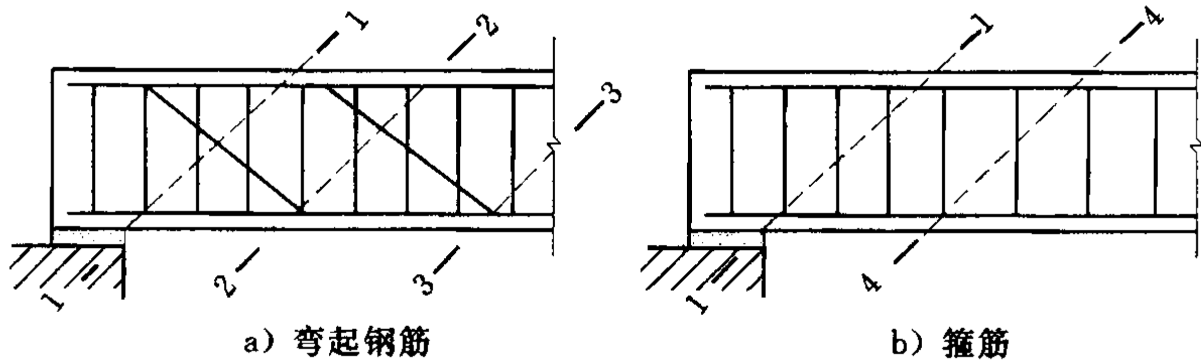
a) 弯起钢筋 b) 箍筋 1—1—支座边缘处的斜截面；2—2、3—3—受拉区弯起钢筋弯起点的斜截面；4—4—箍筋截面面积或间距改变处的斜截面
