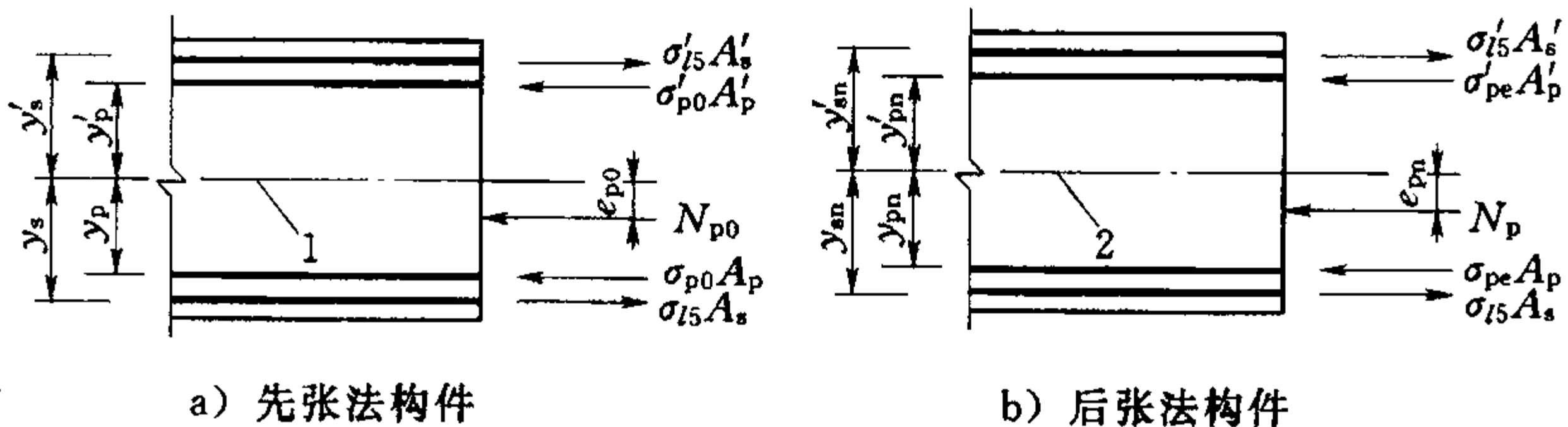
1—换算截面重心轴; 2—净截面重心轴
