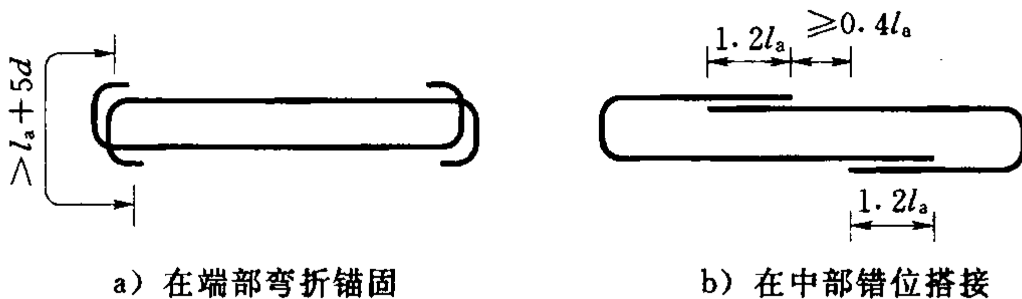
图 10.6.17 分布钢筋的搭接
