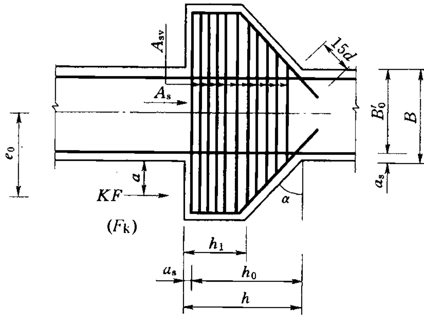
图 10.10.3 中墩弧门支座截面构造
