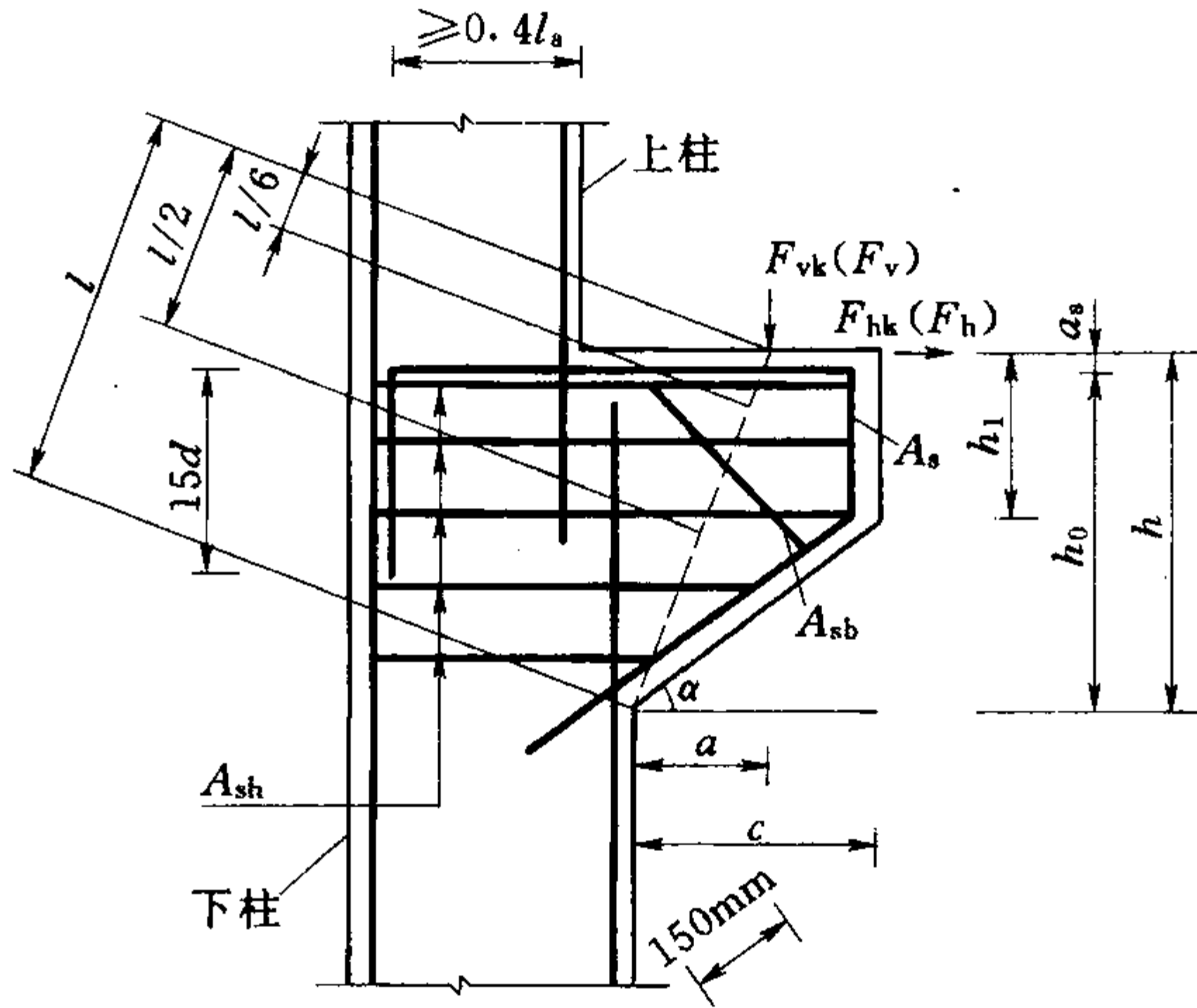
图 10.8.1 牛腿的外形及钢筋布置
