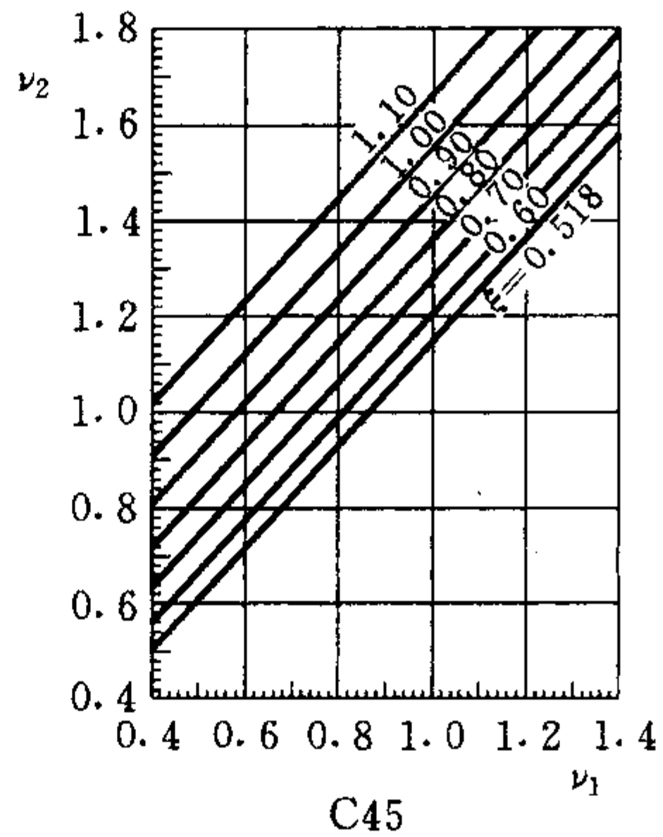
D. 1.3-3 \nu_1 、 \nu_2 与 \xi 关系 (HRB400 级、RRB400 级钢筋 \rho_{\min} = 0.20\% )
