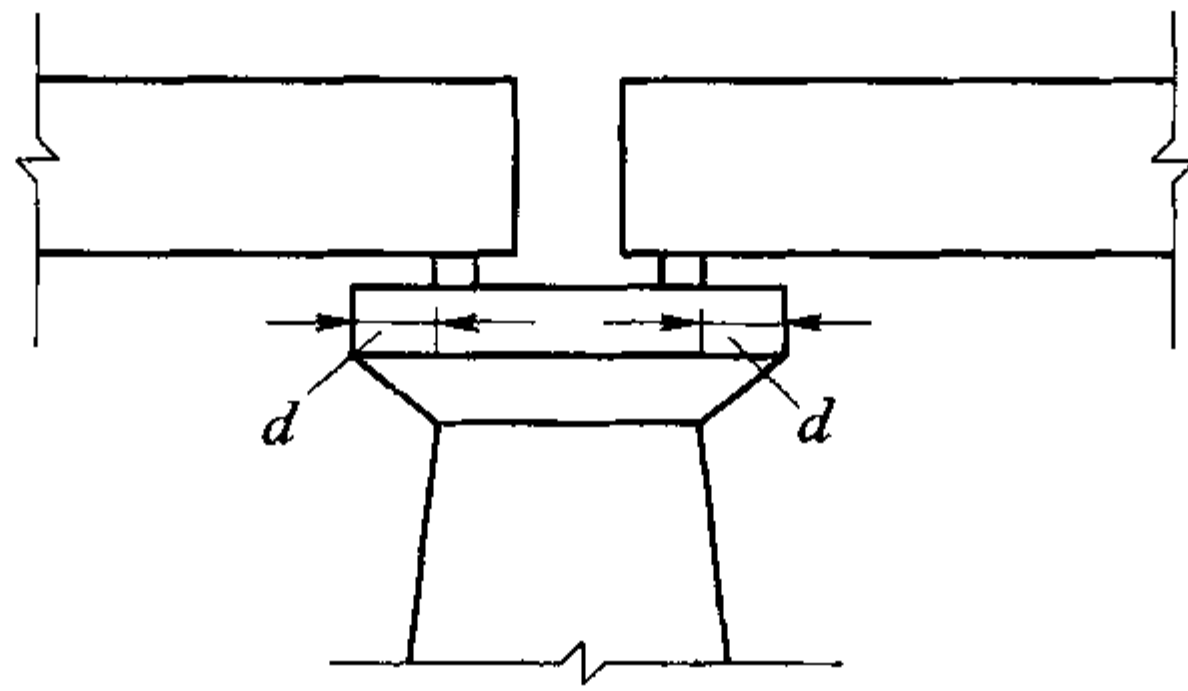
图 13.6.3 支座边缘至墩台帽边缘的距离
