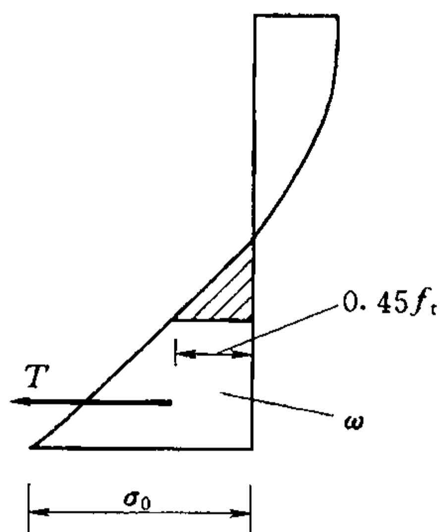
图 12.2.1 按弹性应力图形配筋
