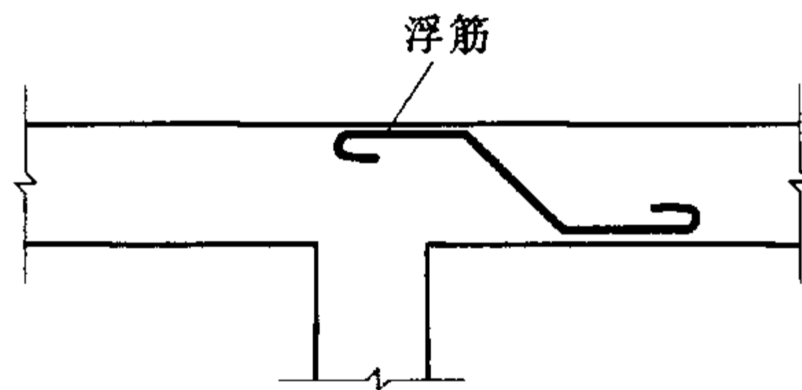
图 1 “浮筋”示意图
