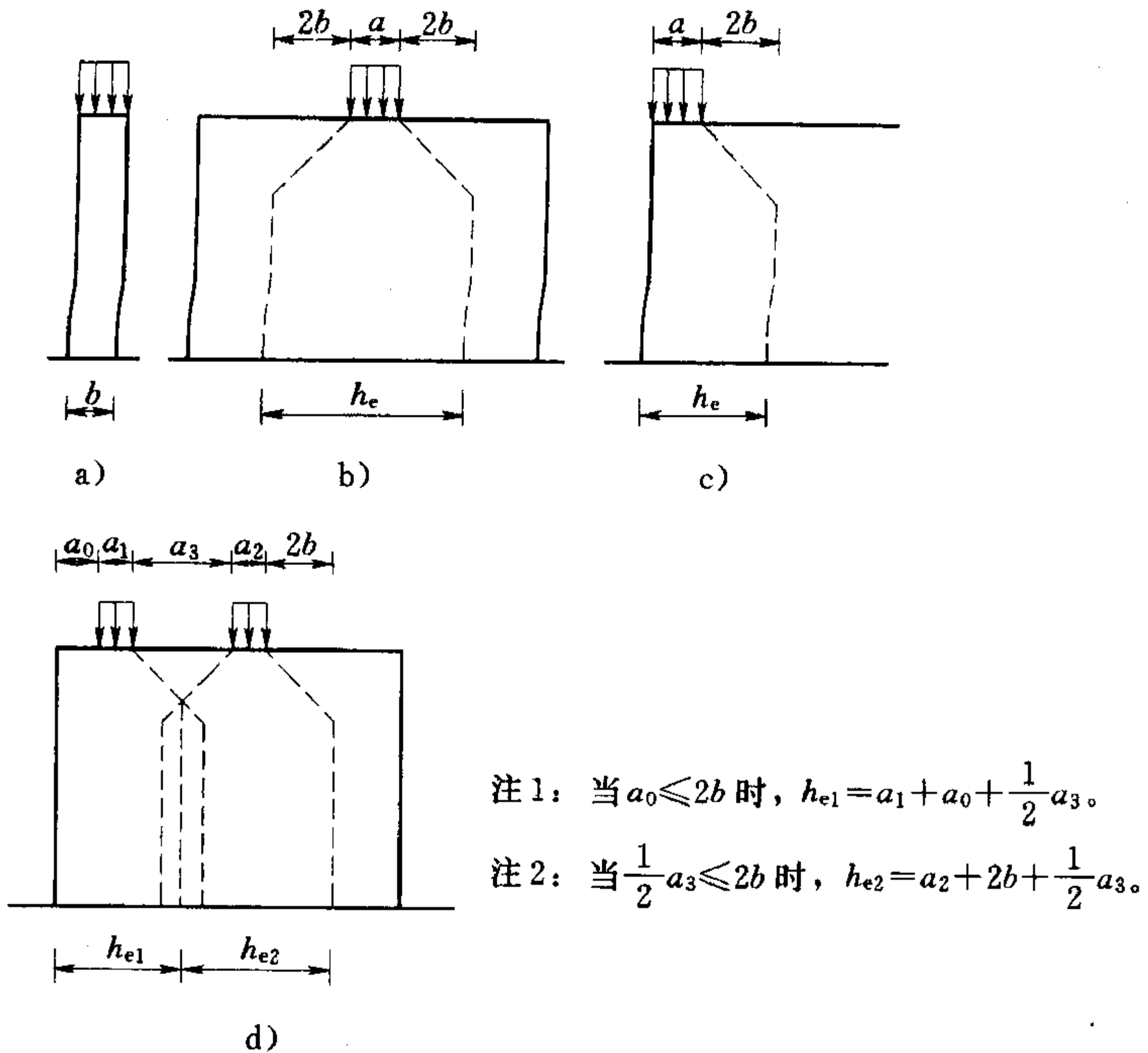
图 10.5.4 墙体有效边长的计算
