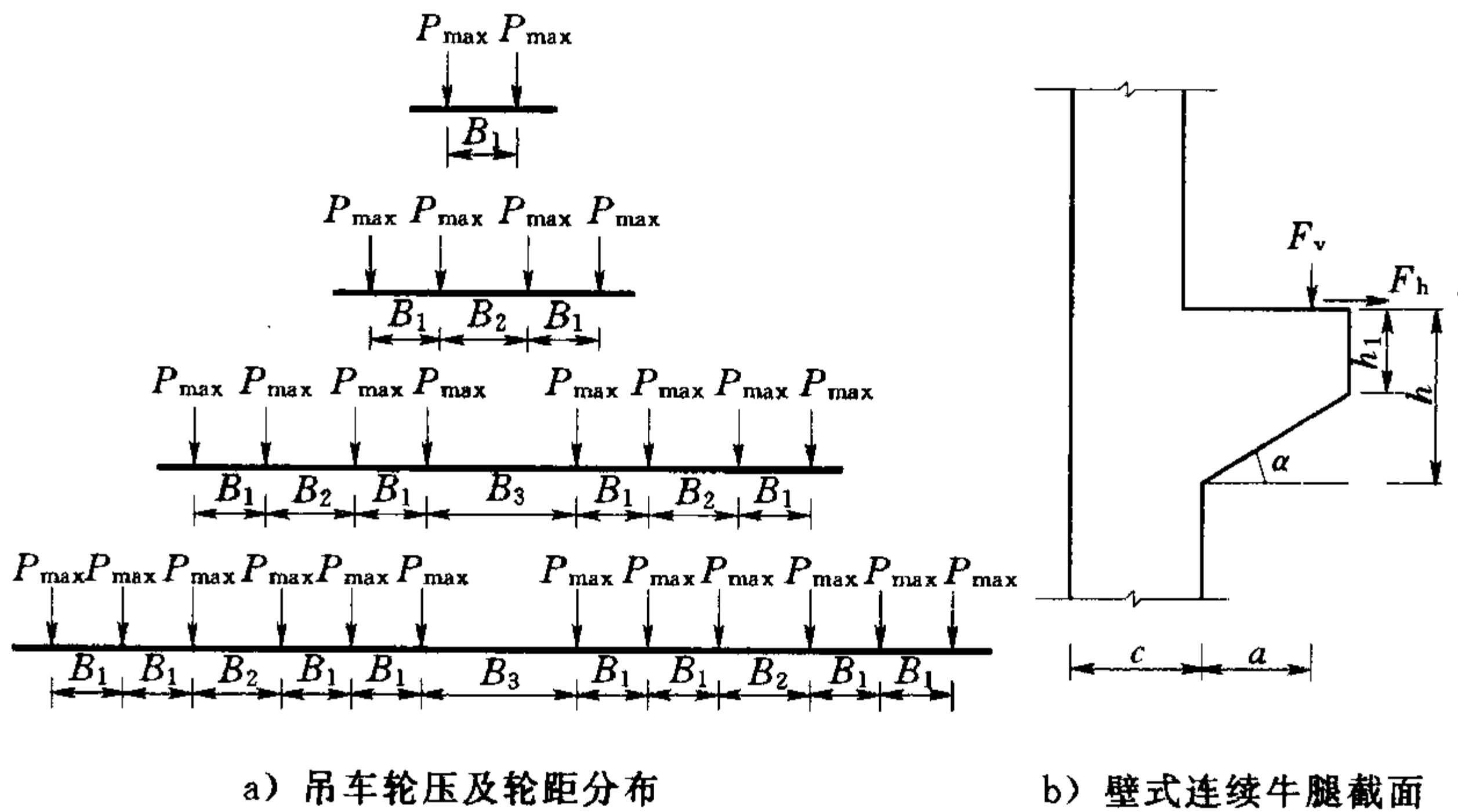
图 10.9.1 壁式连续牛腿轮压分布宽度计算
