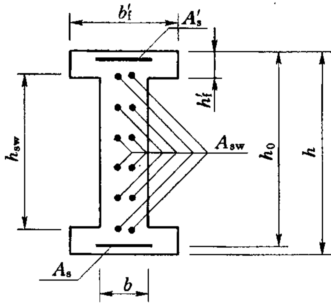
图 6.3.5 沿截面腹部均匀配筋的 I 形截面
