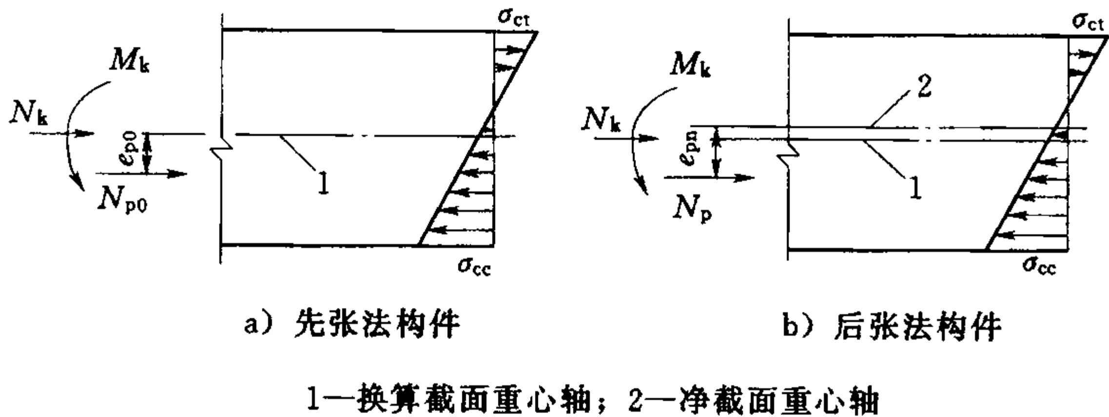
图 8.1.8 预应力混凝土构件施工阶段验算
