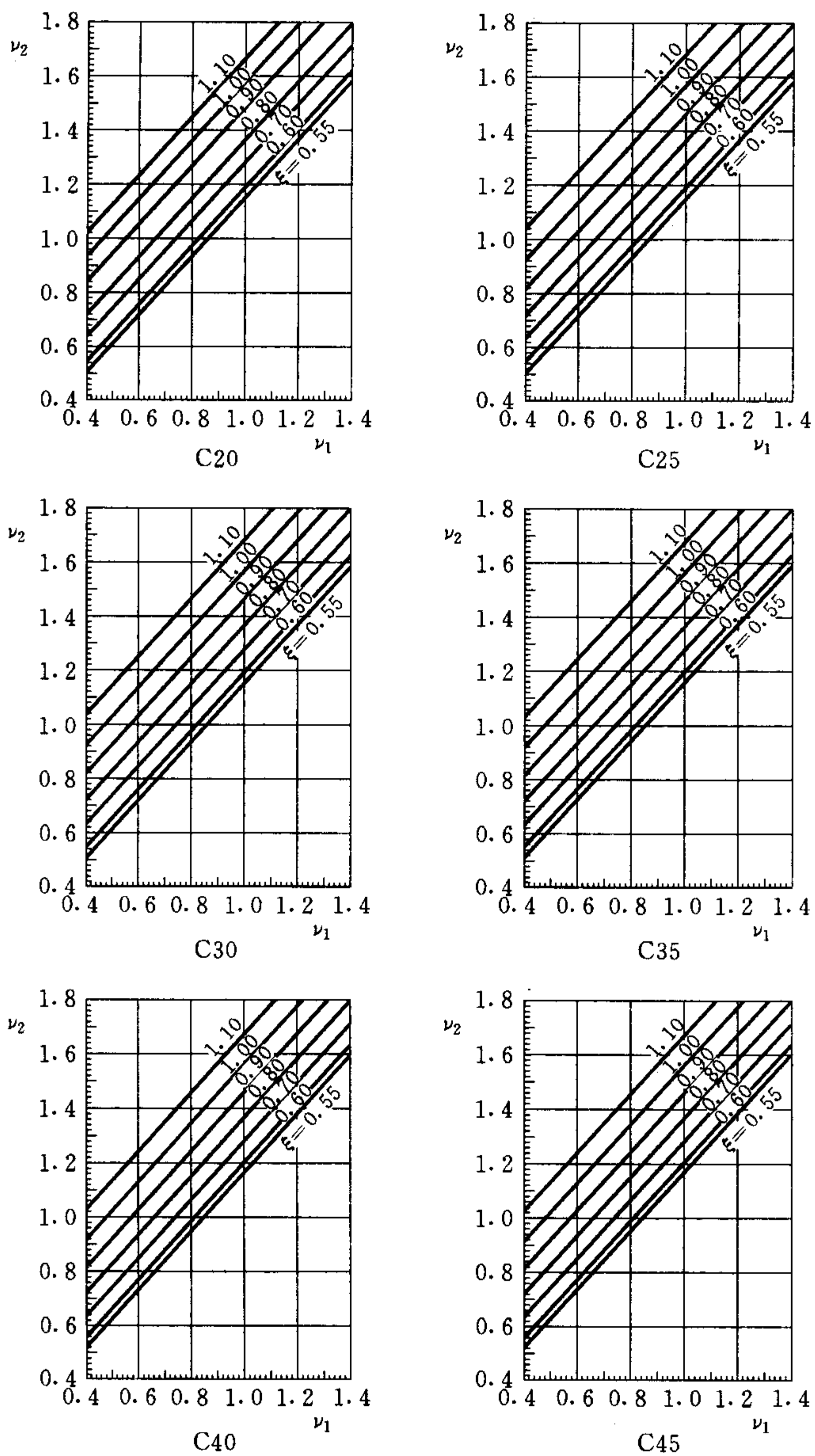
图 D. 1.3-2 \nu_1 、 \nu_2 与 \xi 关系 (HRB335 级钢筋 \rho_{\min} = 0.20\% )
