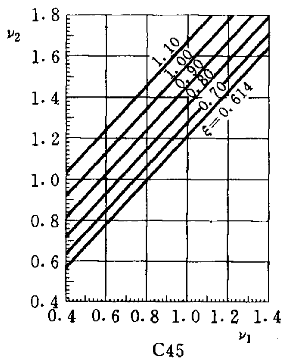
图 D.1.3-1 \nu_1 、 \nu_2 与 \xi 关系 (HPB235 级钢筋 \rho_{\min} = 0.25\% )
