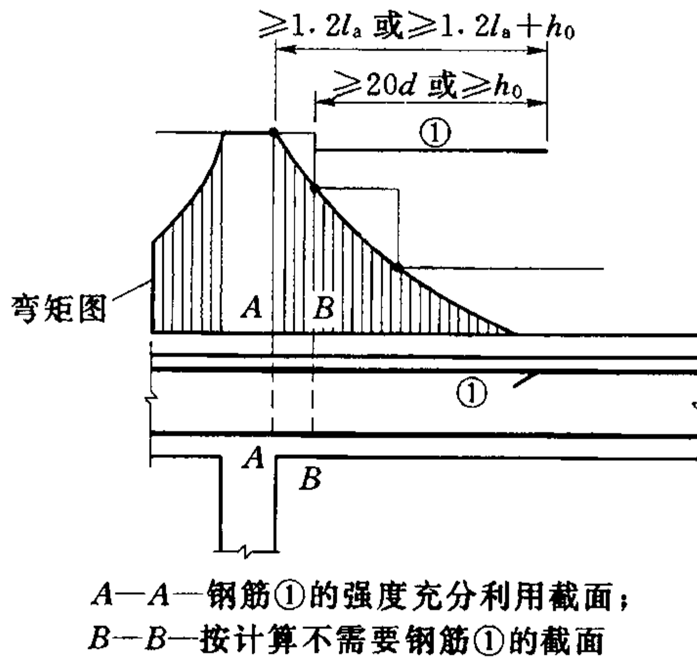
图 10.2.4 纵向受拉钢筋截断时的延长度
