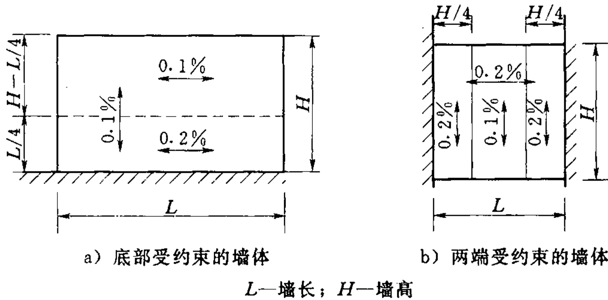
图 11.2.4 墙体温度钢筋配置
