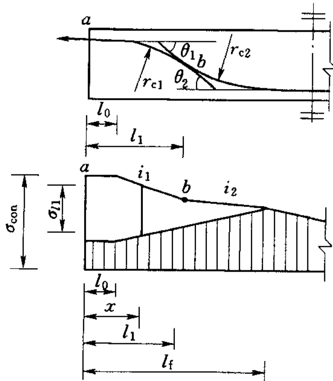
图 E.0.2 两条圆弧形曲线组成的预应力钢筋的预应力损失值 \sigma_{l1}
