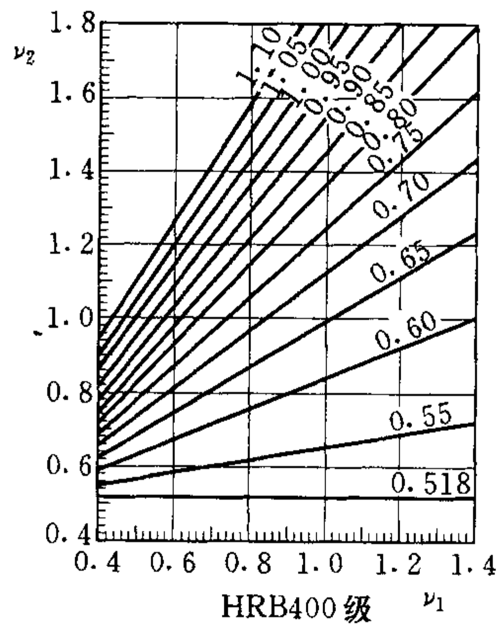
图 D. 2. 1 \nu_1 、 \nu_2 与 \xi 关系
