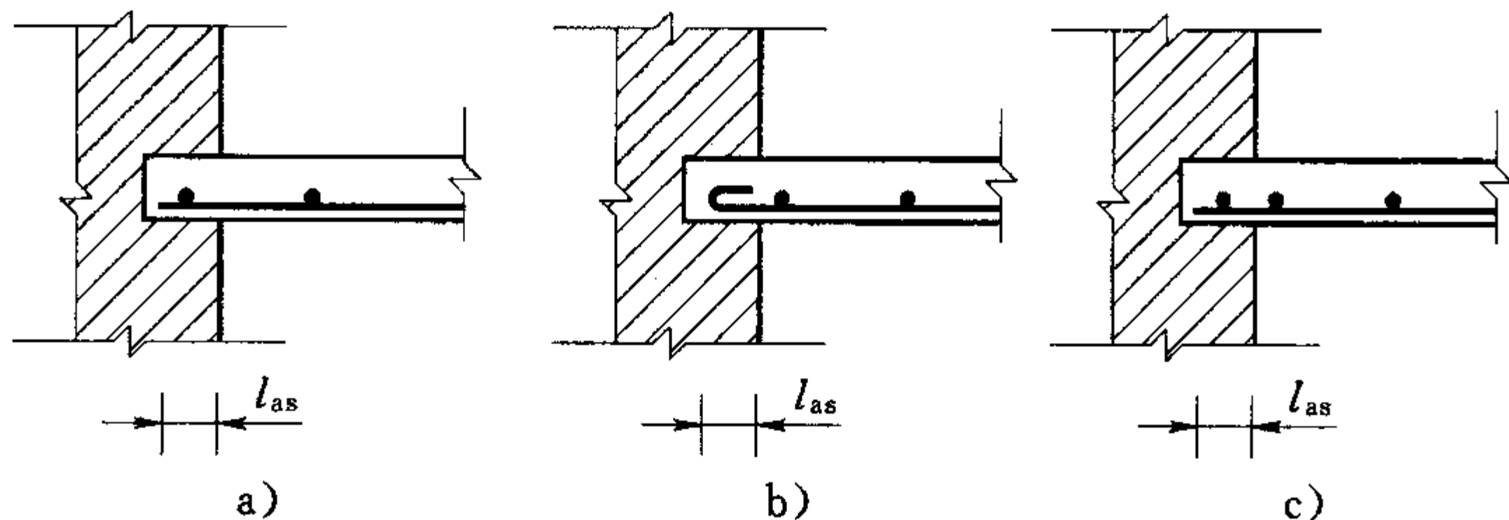
图 10.1.5 焊接网在板的简支支座上的锚固
