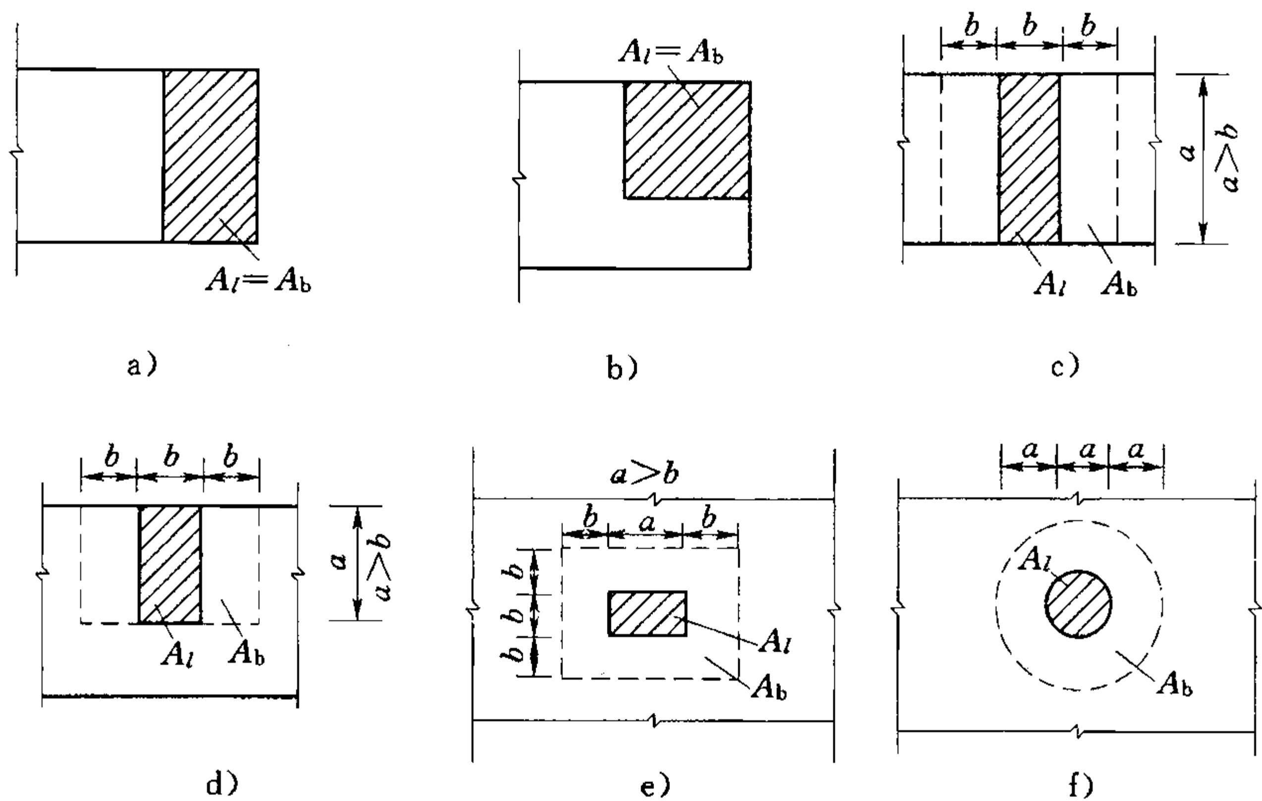
图 5.4.1 确定局部受压计算底面积 A_b
