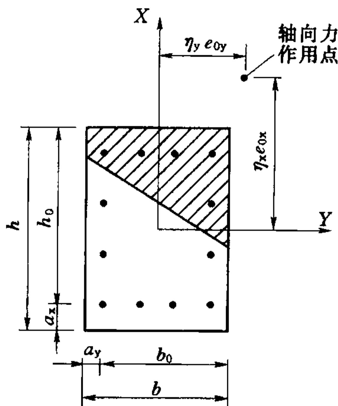
图 6.3.13 双向偏心受压构件的截面
