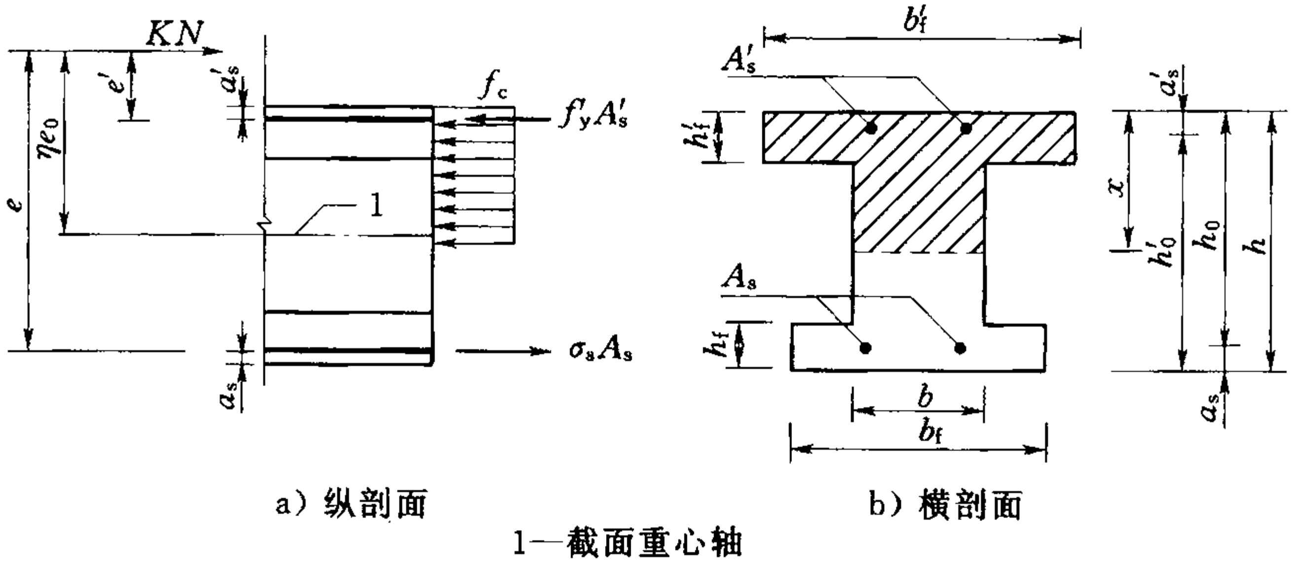
图 6.3.4 I 形截面偏心受压构件的正截面受压承载力计算
