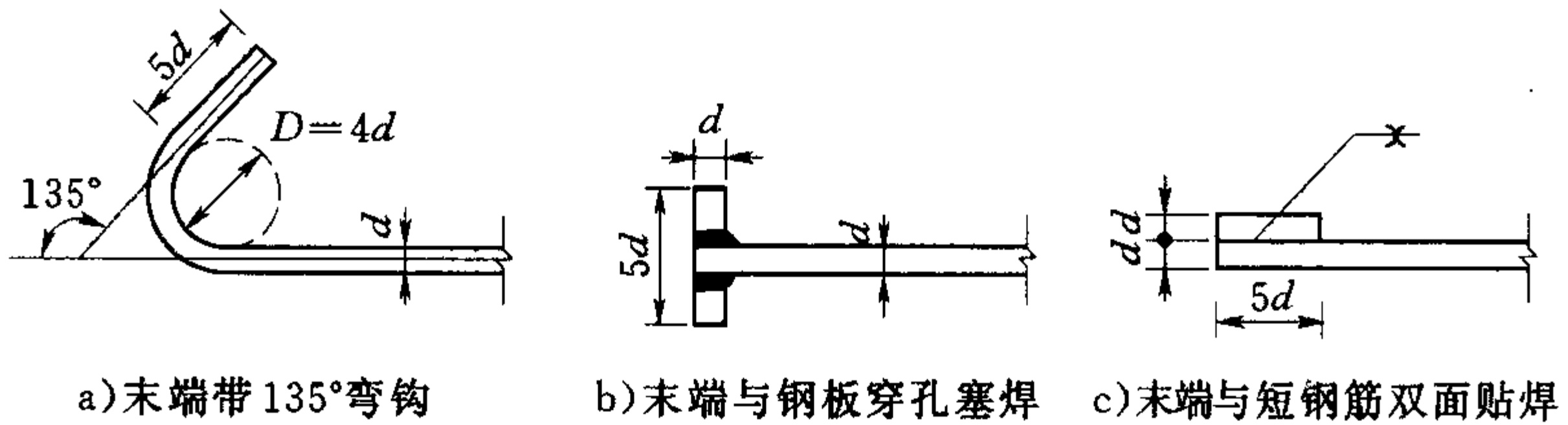
图 9.3.3 钢筋附加锚固的形式及构造要求
