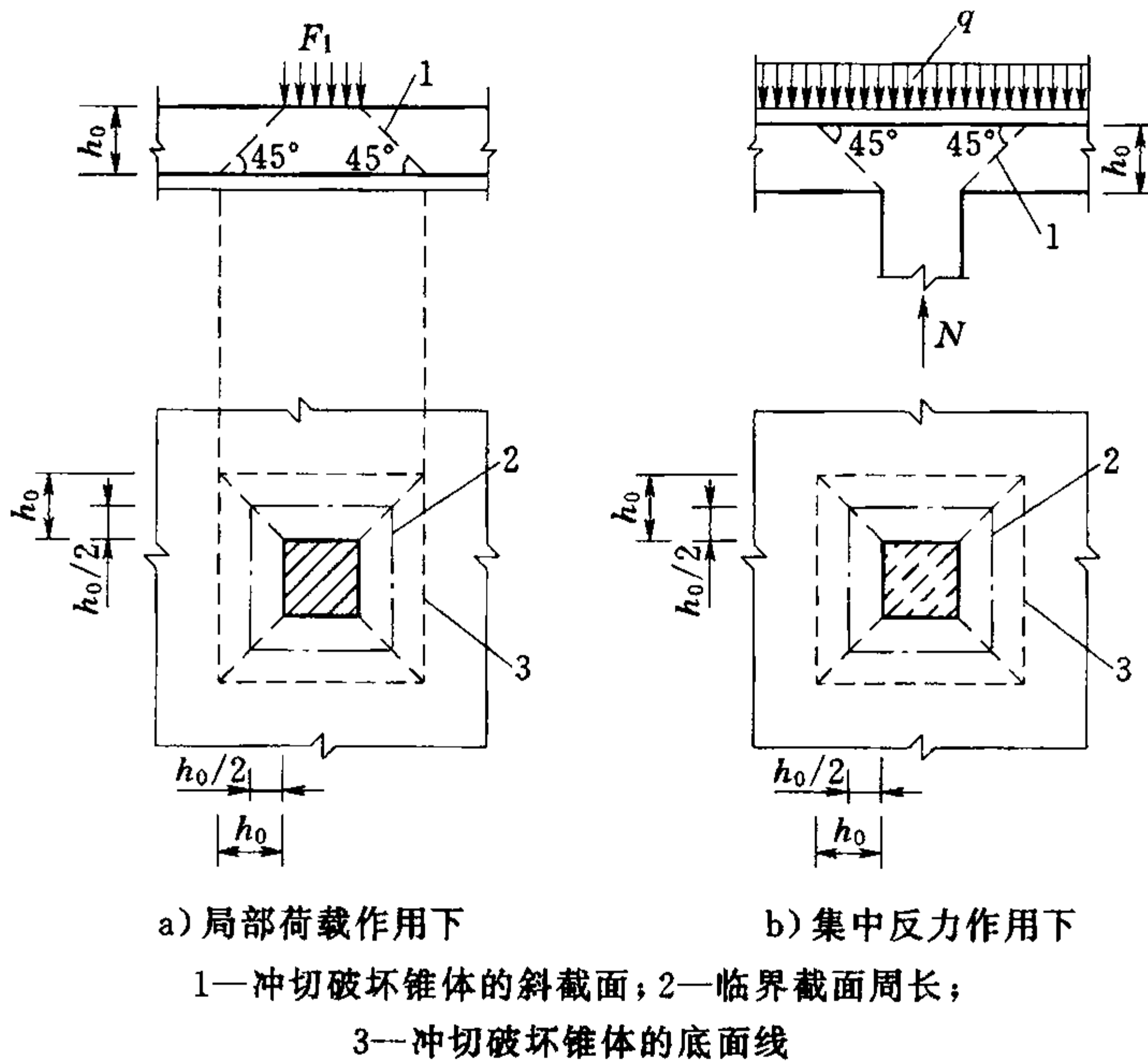
图 6.7.1 板的受冲切承载力计算
