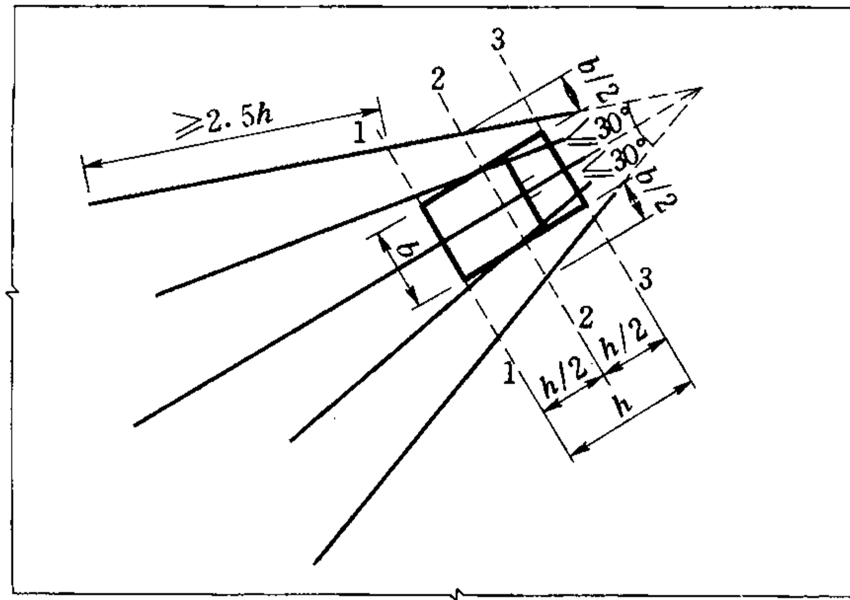
图 10.10.2 闸墩局部受拉钢筋的有效分布范围
