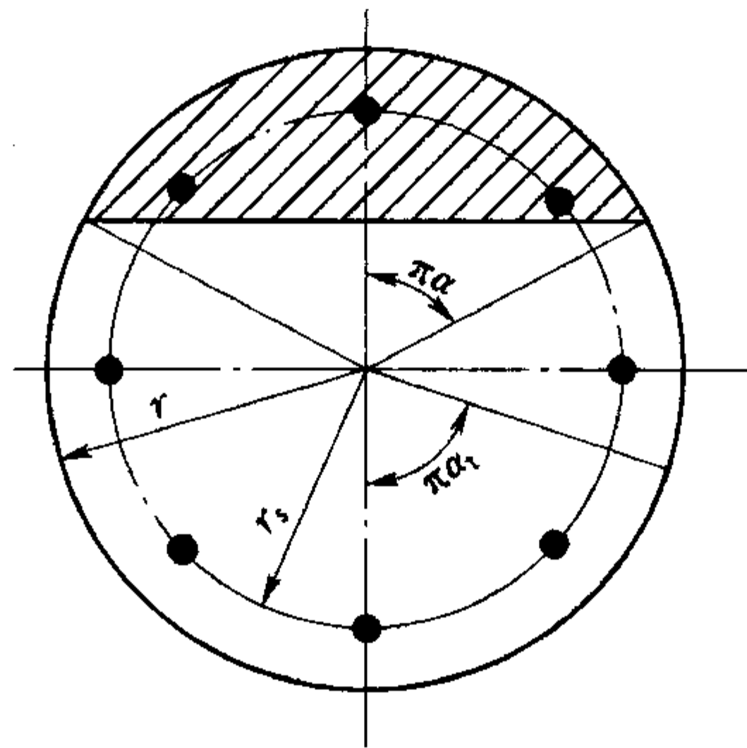
图 6.3.7 沿周边均匀配筋的圆形截面
