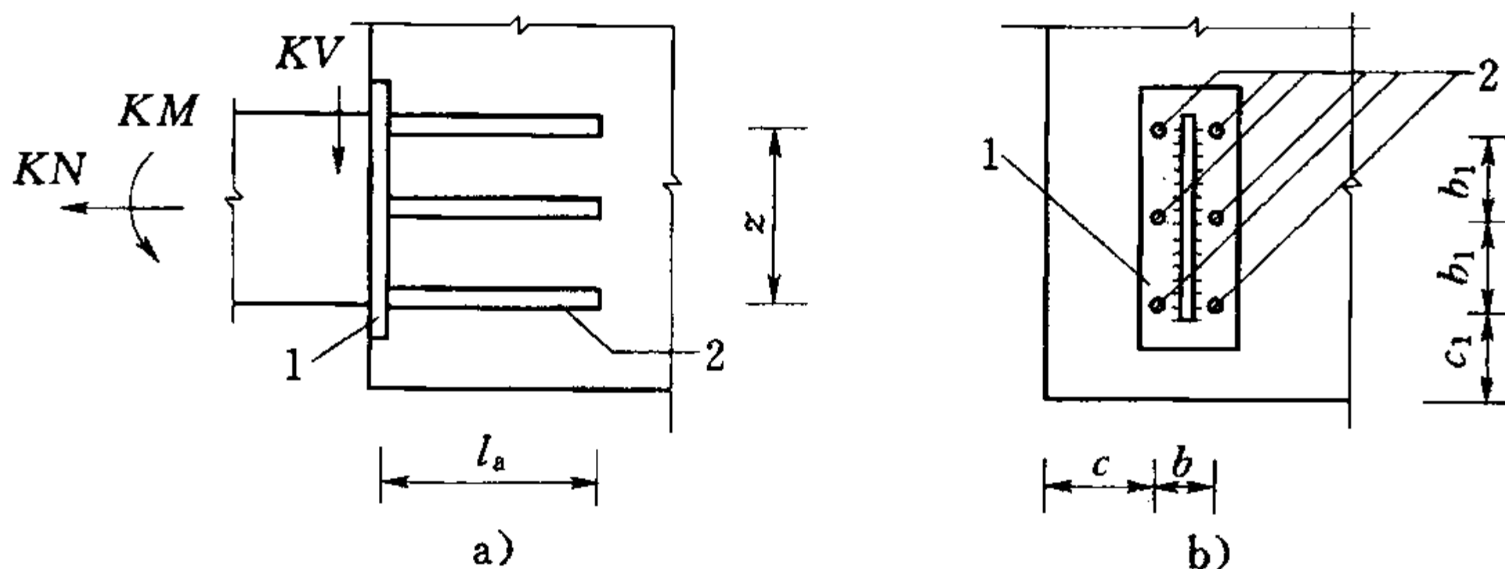
1—锚板；2—直锚筋
