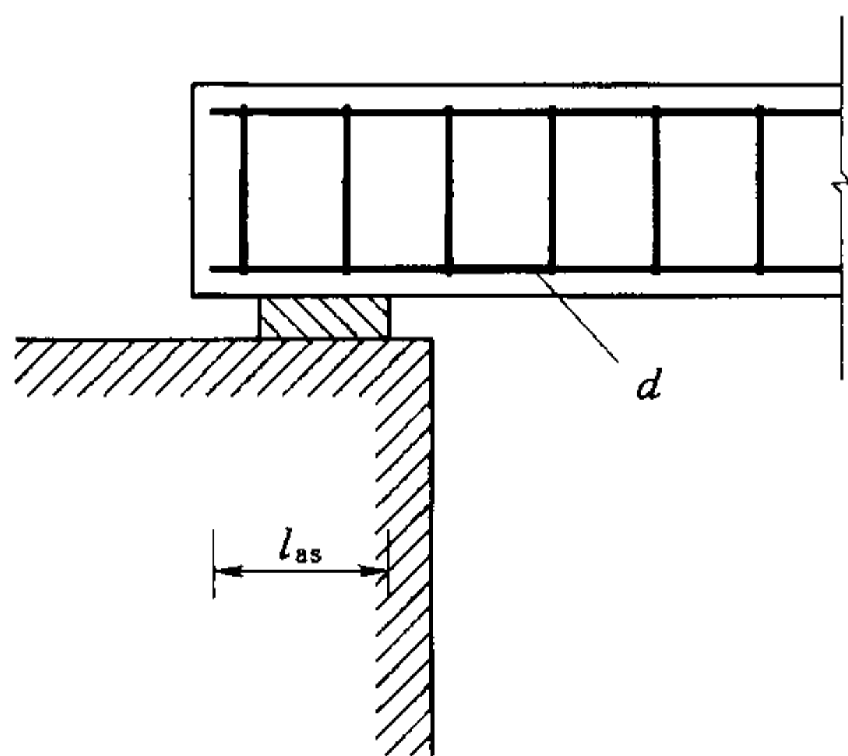
图 10.2.3 纵向受力钢筋在支座上的锚固
