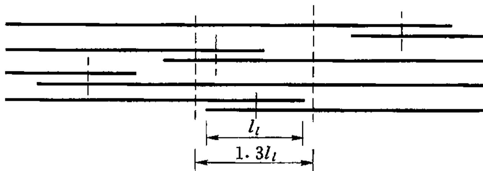
图 9.4.5 同一连接区段内的纵向受拉钢筋绑扎搭接接头
