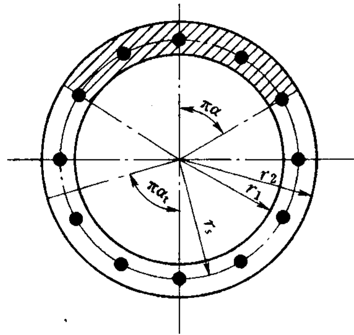
图 6.3.6 沿周边均匀配筋的环形截面
