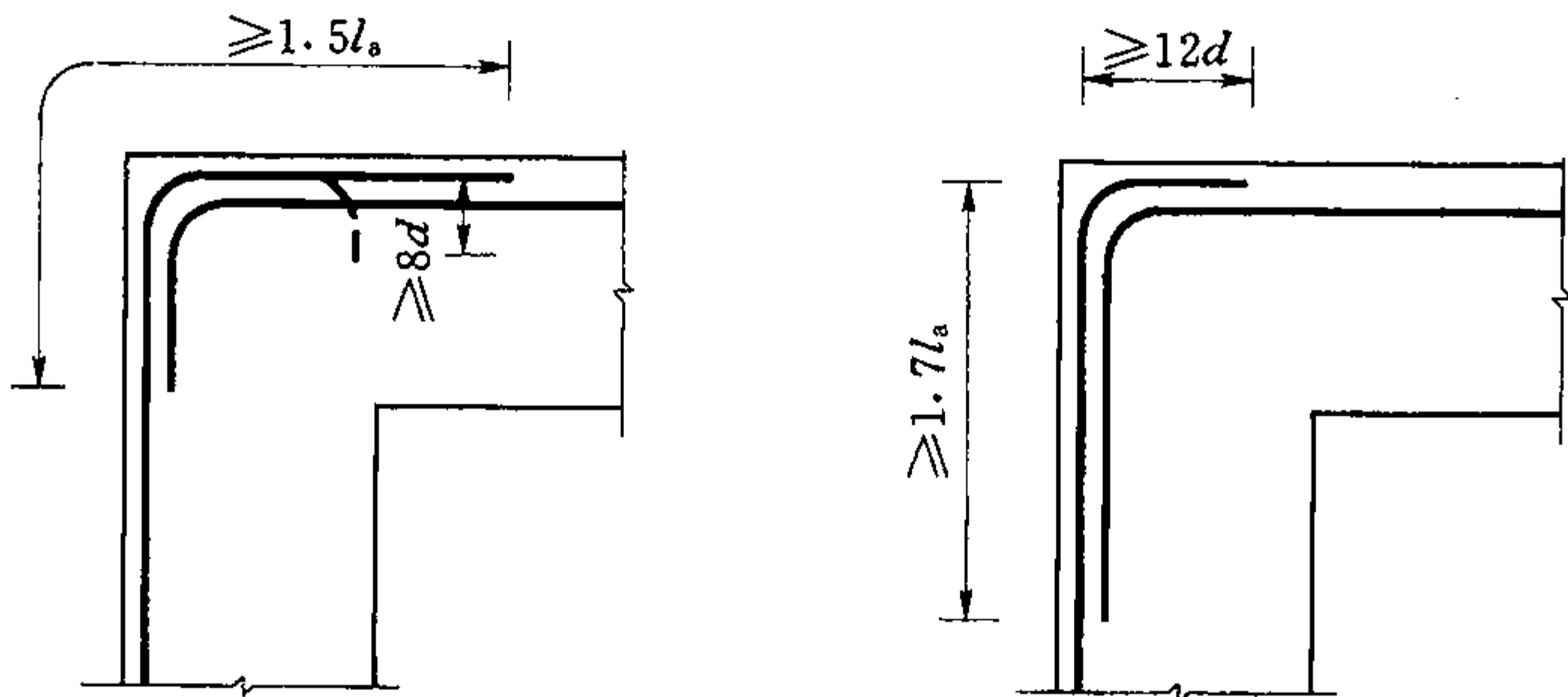
a) 位于节点外侧和梁端顶部的弯折搭接接头 b) 位于柱顶部外侧的直线搭接接头
